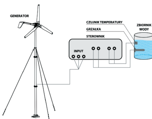
Schemat do podgrzewania c.w.u.
