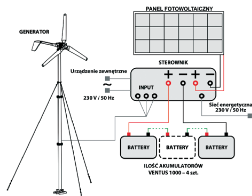
Schemat połączenia - hybryda: wiatrak + panel fotowoltaiczny
