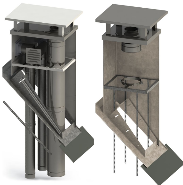
Foto: komin z blachy przekrój
